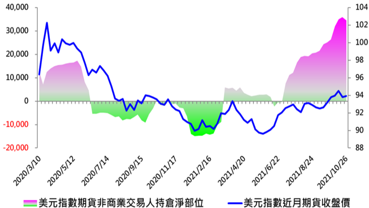
CFTC 美元指數期貨非商業交易人持倉淨部位
